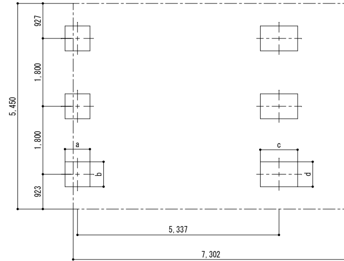
■ 基礎配置図
